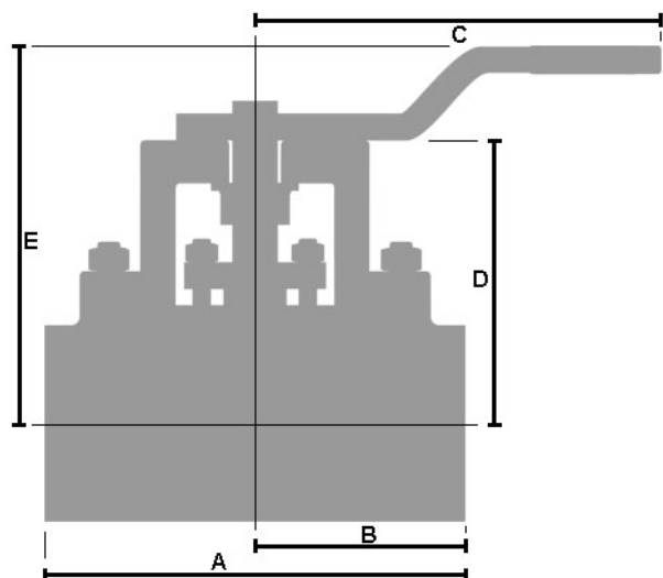
Wymiary zaworów RSVP klasy 3100
